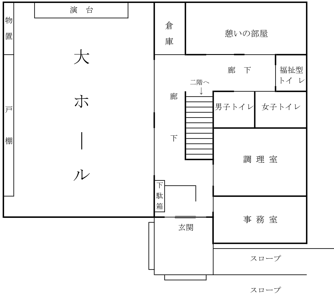
(1階平面図)
